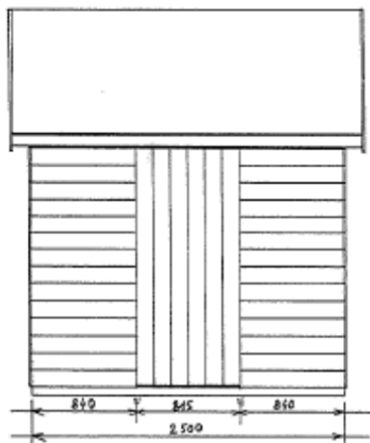
CHALET DE NOËL DE 5.40m x 2.50m
