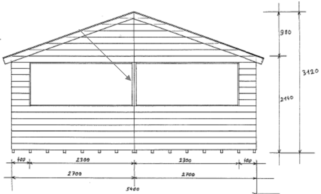
CHALET DE NOËL DE 5.40m x 2.50m
