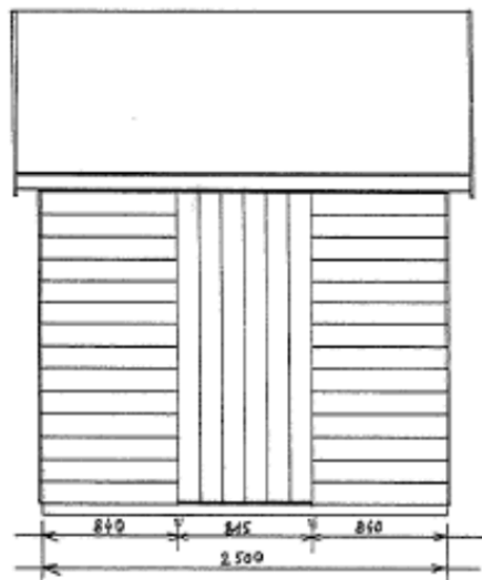
CHALET DE NOËL DE 5.40m x 2.50m
